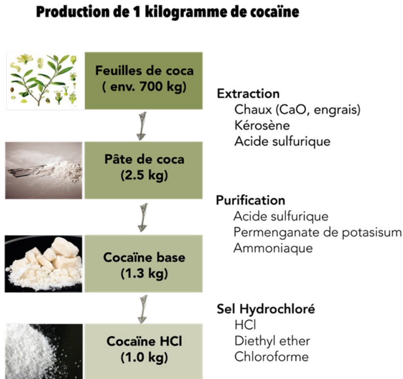
Figure 2 Processus de fabrication de la cocaïne
