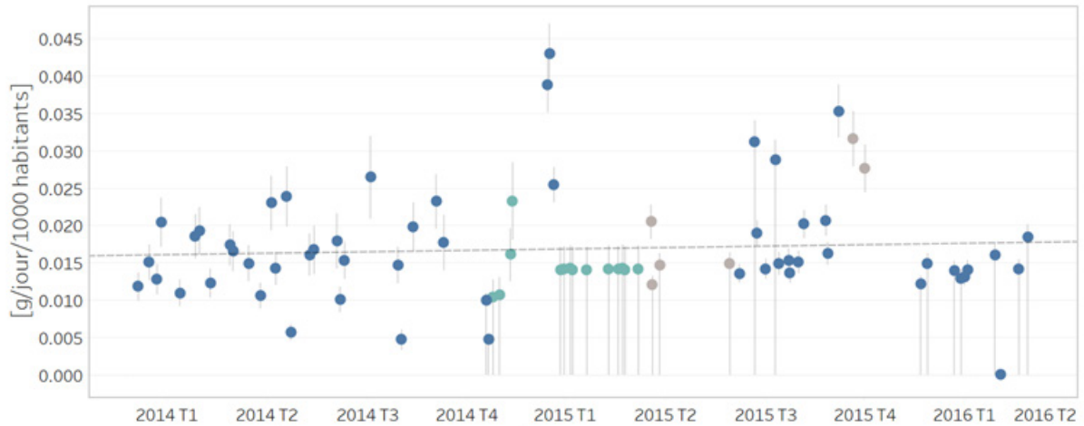
Figure 40 Evolution des quantités de méthamphétamine pure consommée en région lausannoise de 2014 à 2016
