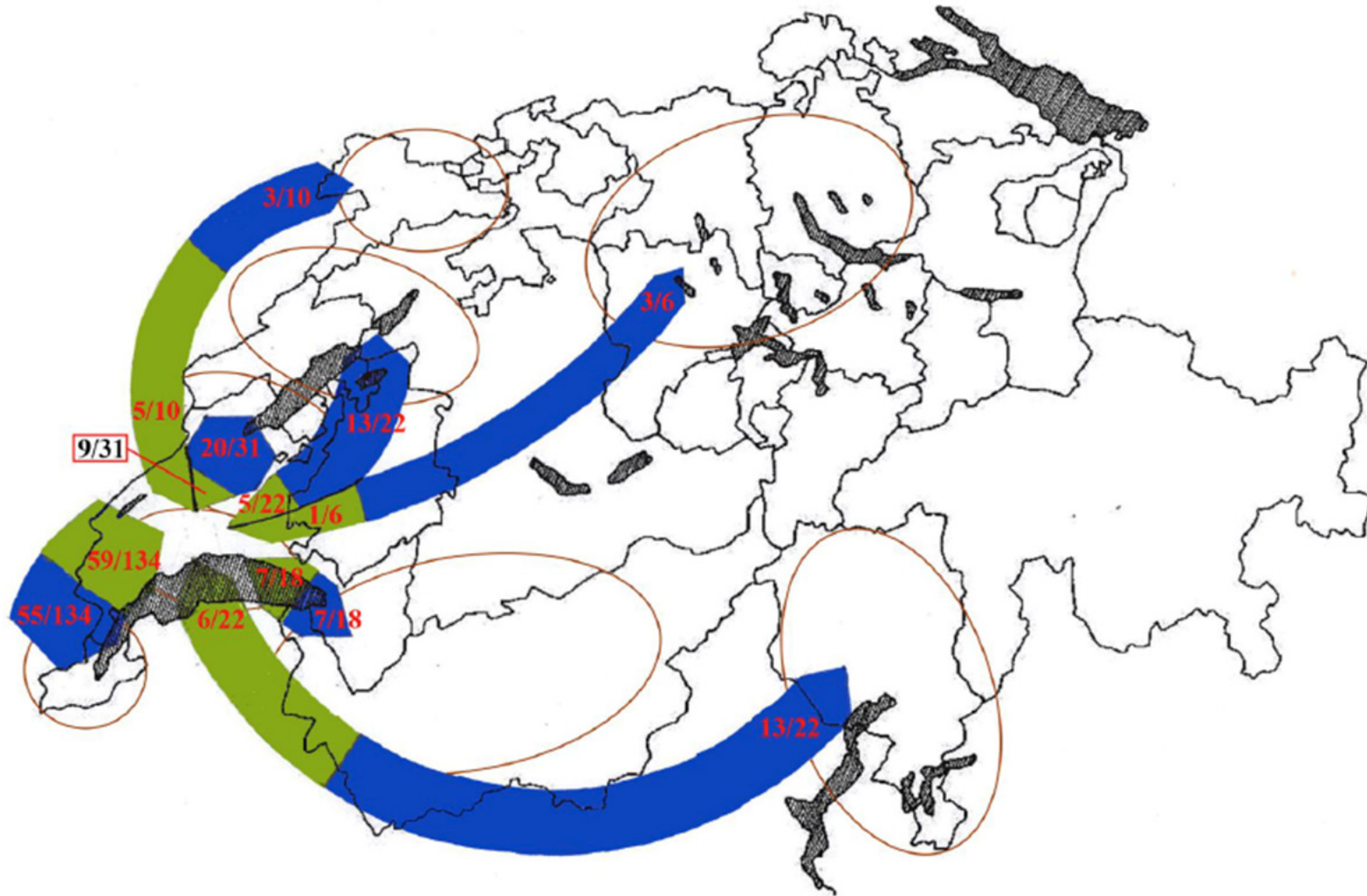
Figure 15 Dynamique spatiotemporelle des classes chimiques de 2006 à 2015 pour les saisies de cocaïne par rapport à la zone « Lausanne »*.
