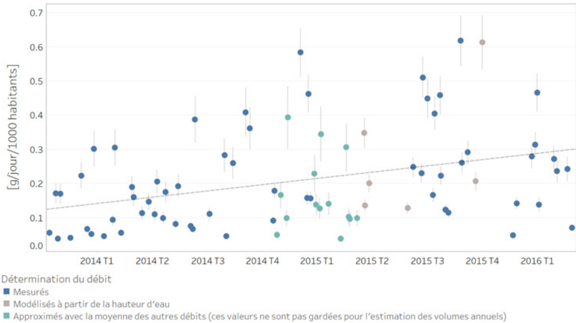
Figure 30 Evolution des quantités de MDMA pure consommée en région lausannoise de 2014 à 2016
