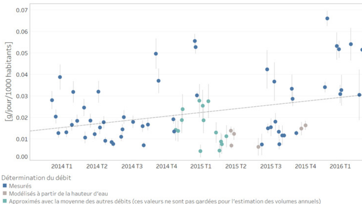
Figure 35 Evolution des quantités d'amphétamine pure consommée en région lausannoise de 2014 à 2016
