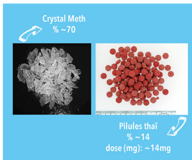
Figure 37 Principales formes et puretés moyennes de la méthamphétamine analysée par les laboratoires associés à la SGRM (spécimens saisis entre 2014 et 2016)
