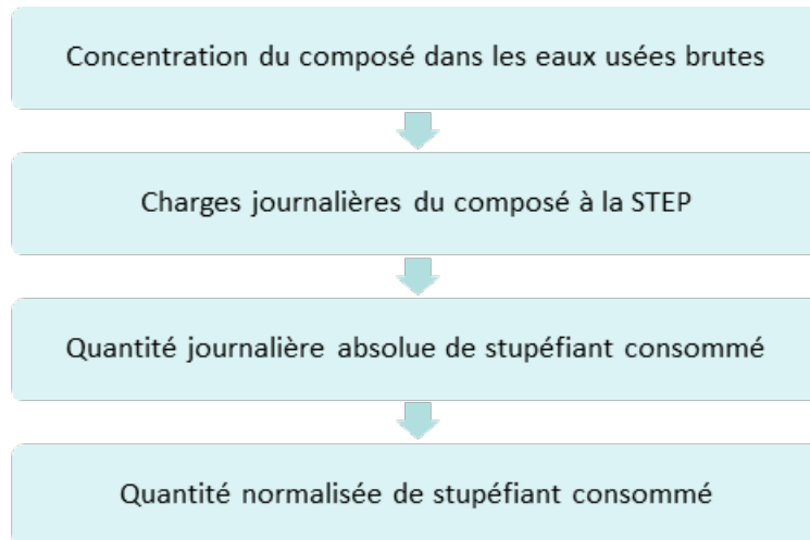
Figure 20 Etapes principales des estimations de volumes par l'analyse des eaux usées
