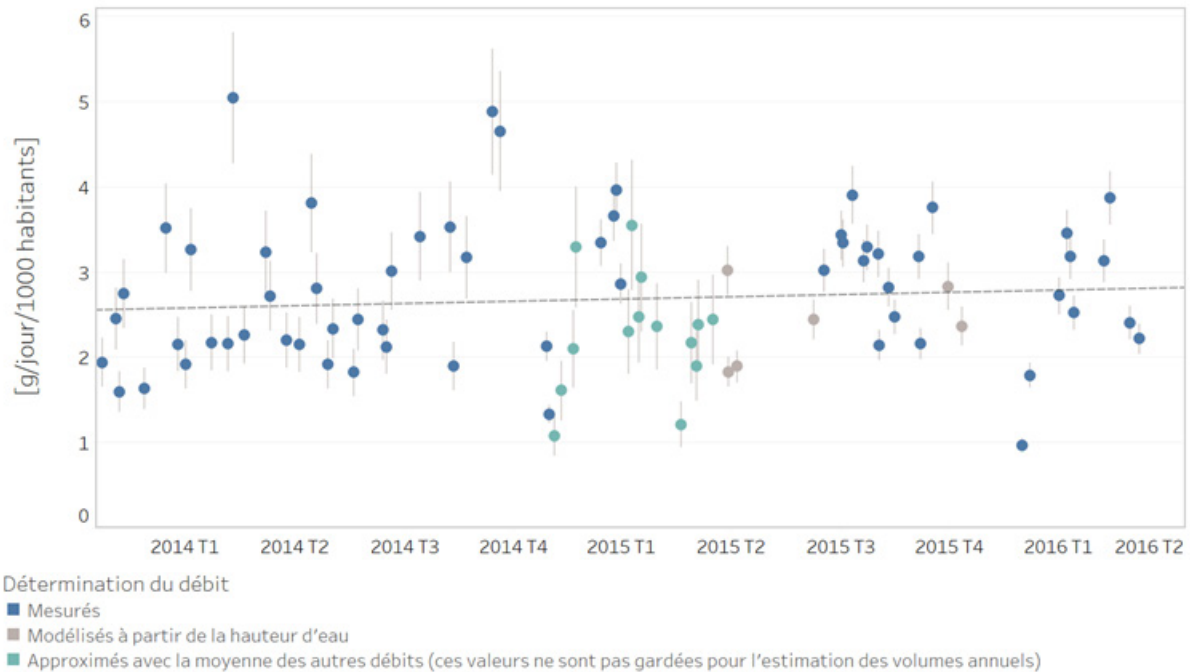
Figure 23 Evolution des quantités de cocaïne en tenant compte de sa pureté au niveau de la consommation en région lausannoise de janvier 2014 à mai 2016
