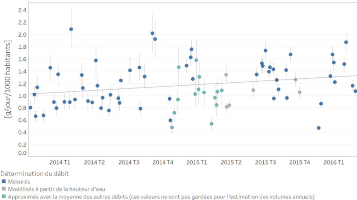
Figure 22 Evolution des quantités de cocaïne pure consommées en région lausannoise de janvier 2014 à mai 2016 – quantités normalisées par le nombre d’habitants
