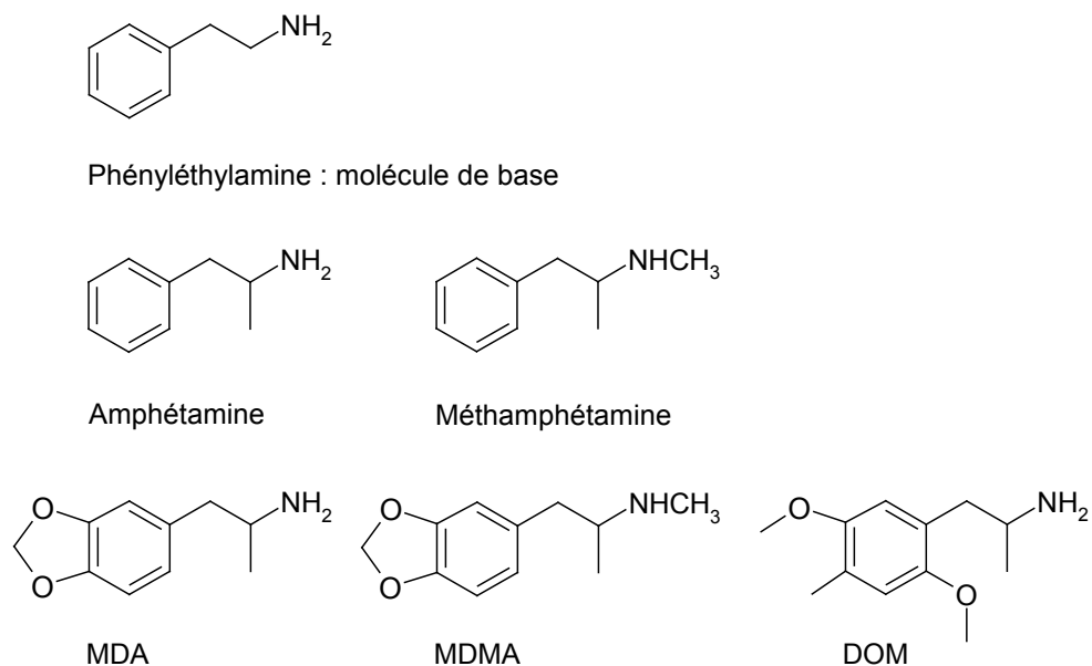
Figure 26 Structure chimique des produits amphétaminiques et dérivés
